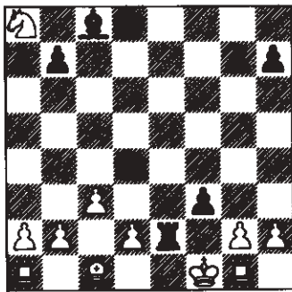
22. Tg1
