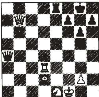
39. ..., Lb6
