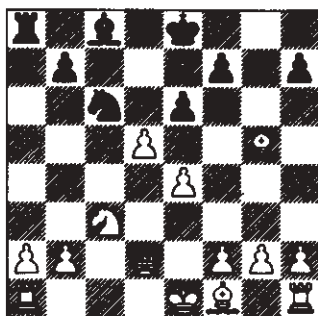
8. Dd2
