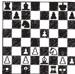
11. Dg3
