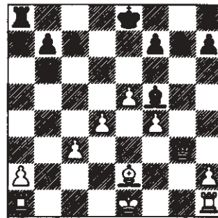
17. d3-d4
