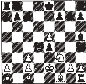
10. ..., Lh5
