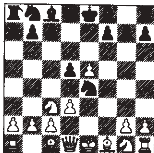
5. d3!?
